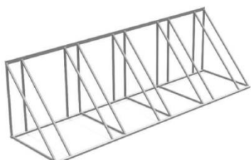
Велопарковка 5-ти местная "Гарби" Размеры: 2500x800x800 мм. Цена: 24 000 р.
